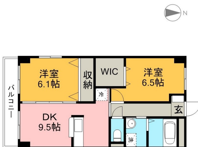
【間取り図】
